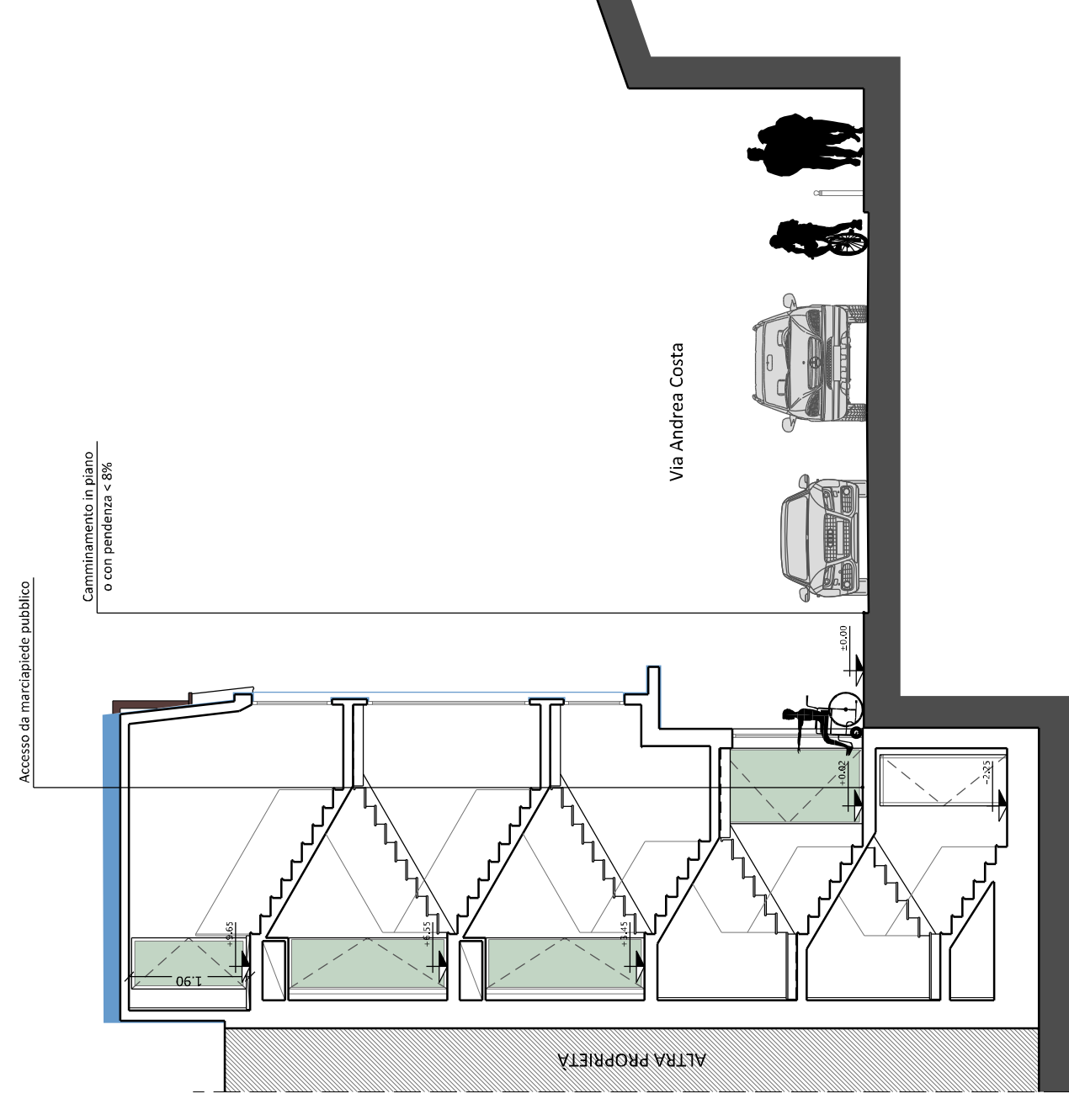
Sezione A-A' _ Sc. 1:100
