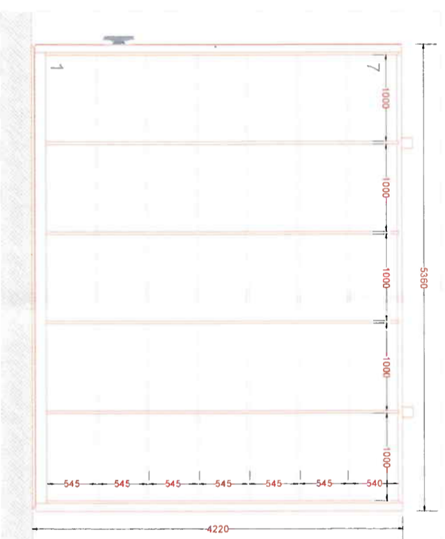
SEZIONE - scaffalatura mobile A
