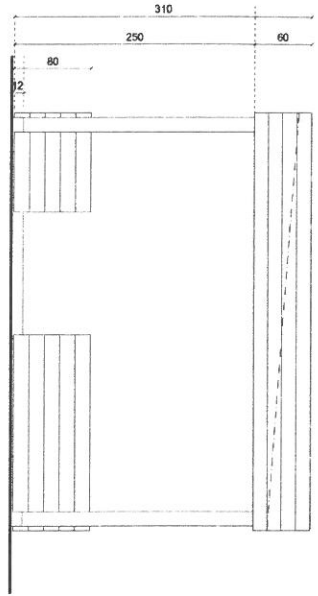
PROSPETTO B-B'
